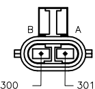
MOTOR PKRD 480 SER SEALED CONN: 1205 2613 (2F) TPA: 1205 9897 TERM: 1205 2139 (10 GA) SEAL: 1203 4170 (10 GA)
